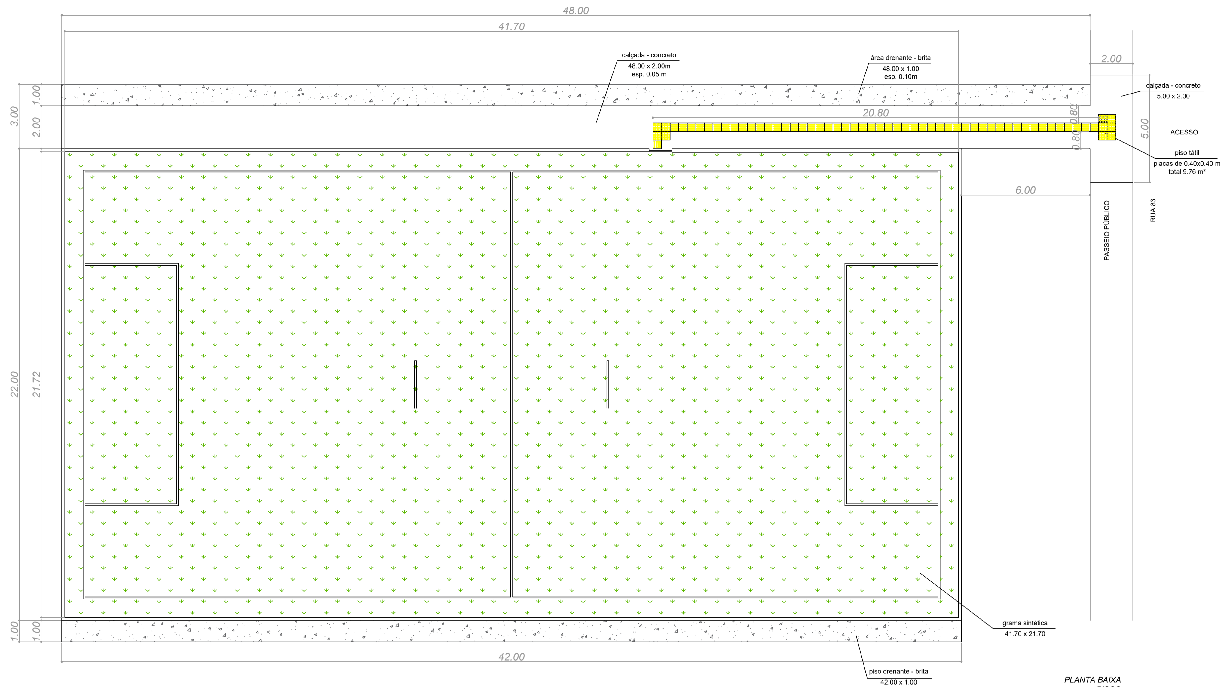
PLANTA BAIXA PISOS ESC.: 1/100
