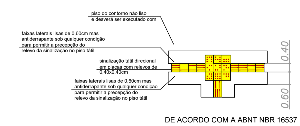
DETALHE DO PISO TÁTIL SEM ESC
