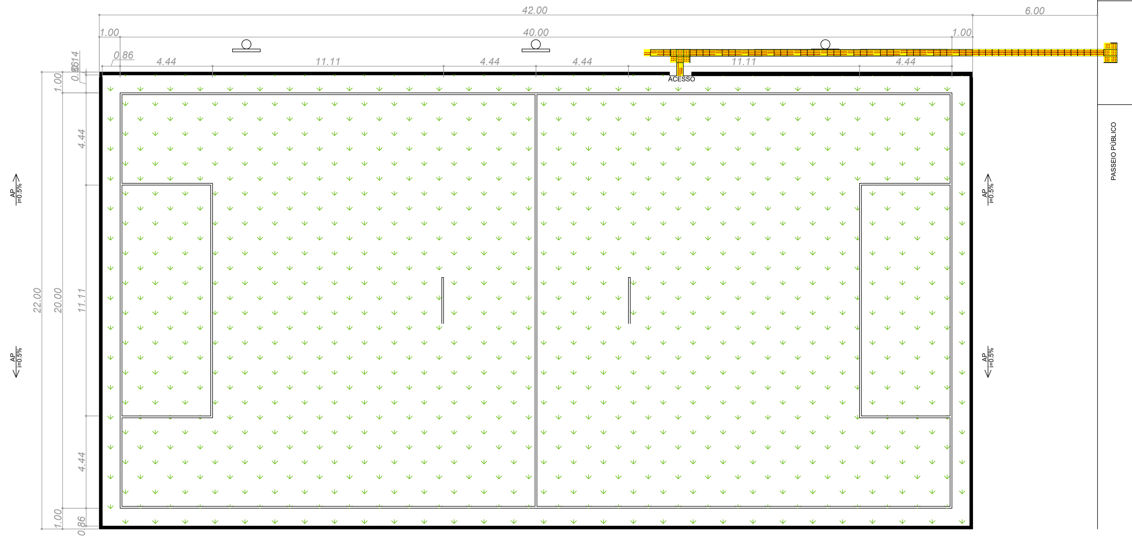
PLANTA BAIXA CAMPO DE FUTEBOL SOCIETY ESC.: 1/100
