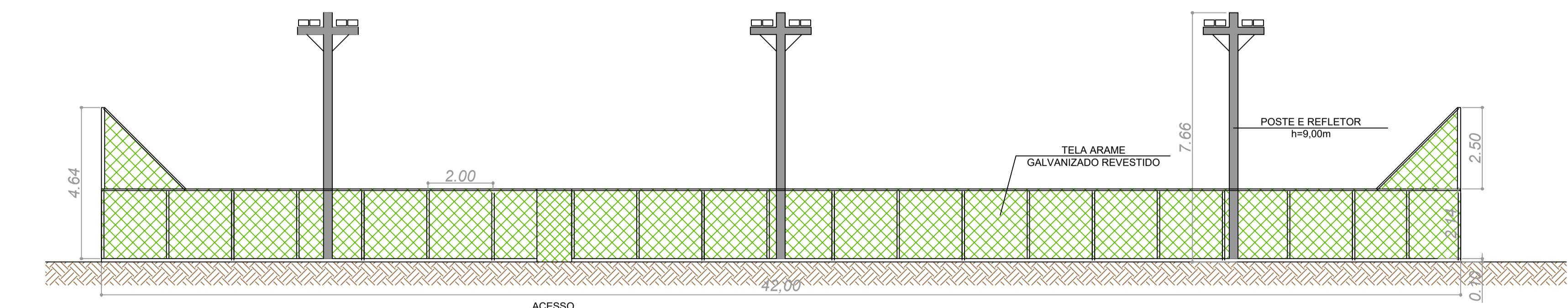
VISTA LATERAL ESC.: 1/100
